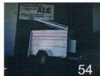
Remolque caja cerrada 2300 x 1300 x 1300 + tapa Eje 1350 Kg C/F Todoterreno conjunto 235/75R15 Cajón delantero
